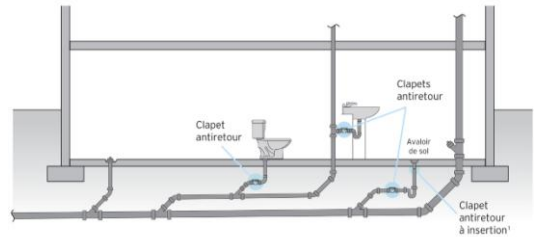
Clapets installés sur les bras de siphon des appareils
