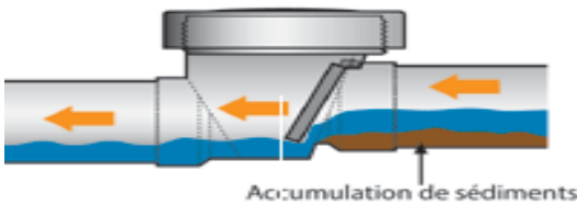
Clapet normalement ouvert
