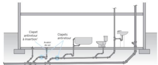
Clapets installés sur les bras de siphon des appareils
